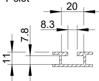
T-Nut/ T-slot
