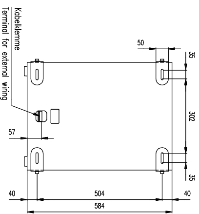
Rückansicht / Rear view Variante 3 / Variation 3
