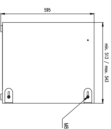
Rückansicht / Rear view Variante 4 / Variation 4
