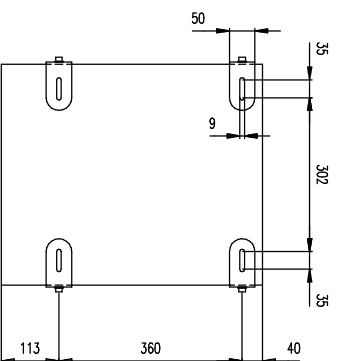
Draufsicht / Top view Variante 1 / Variation 1
