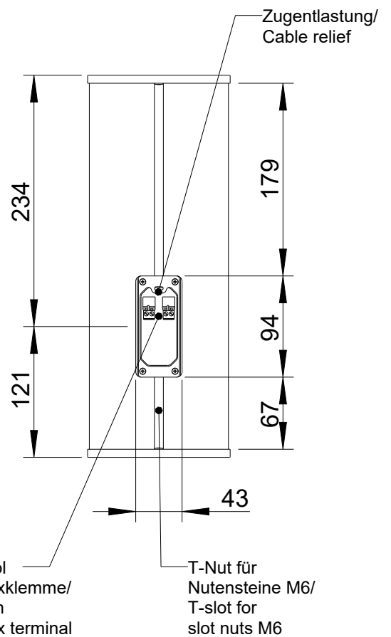
Rückansicht/ Rear view
