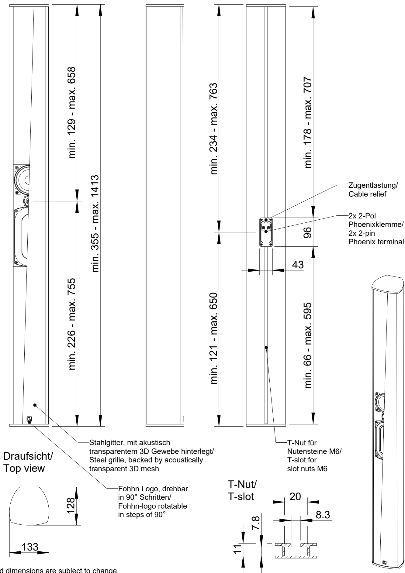
Vorderansicht/ Front view
