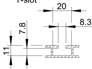
T-Nut/ T-slot
