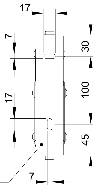
Rückansicht/ Rear view
